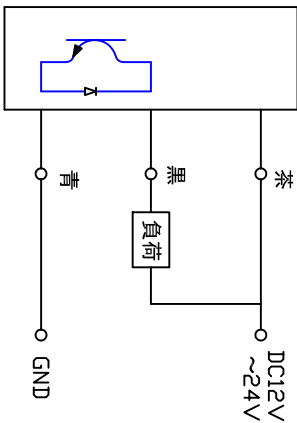
結線図
